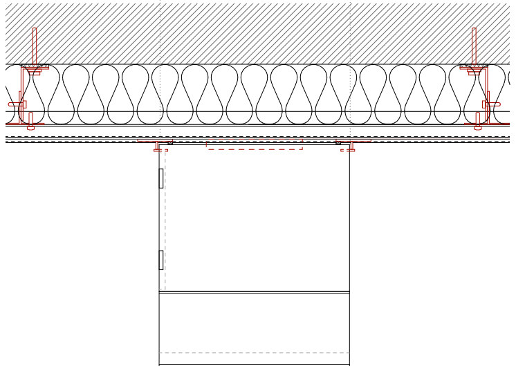
Plan 1:20
