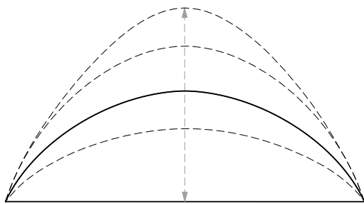
simple parabolas
